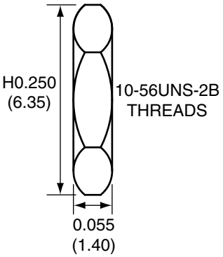
NUT
